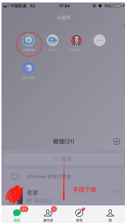
图9 打开小程序
