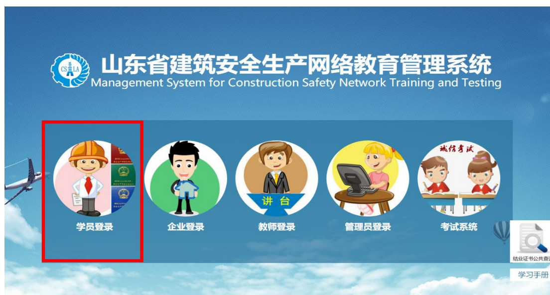
图 3-1 网站首页
